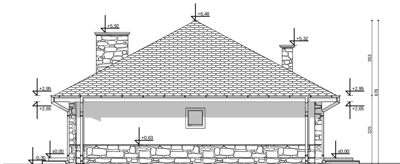
ELEVACJA BOCZNA
