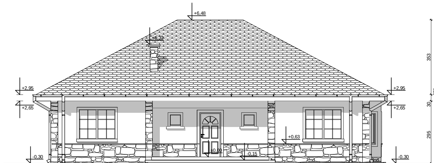
ELEWACJA FRONTOWA
