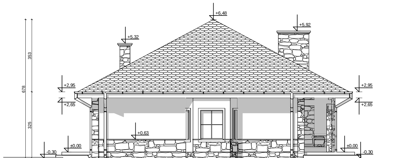
ELEVACJA BOCZNA
