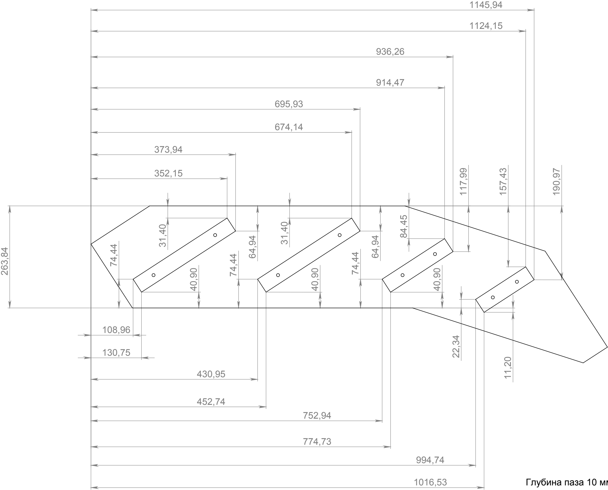
Тетива №2 разметка пазов под ступени
