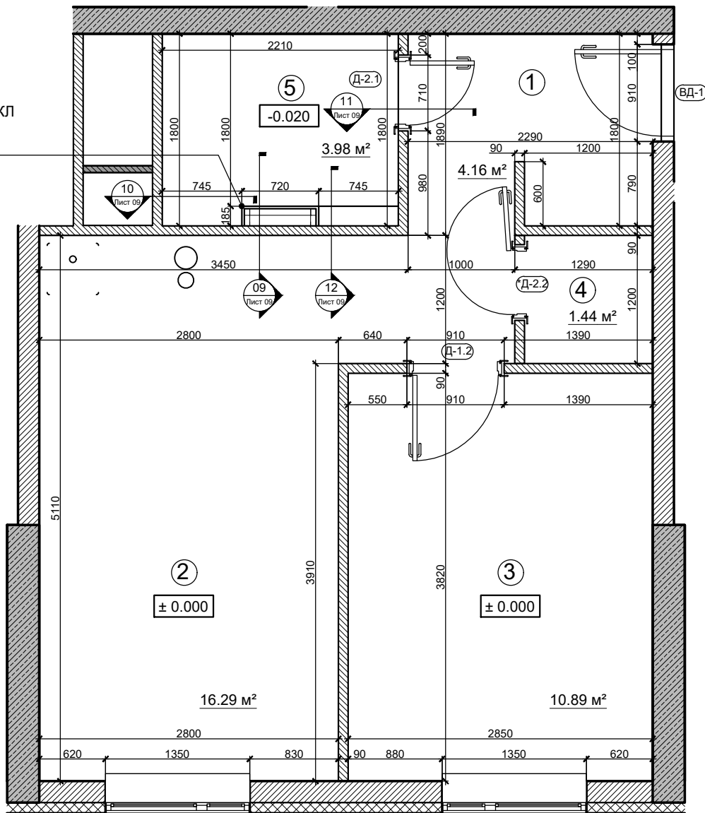
ПЛАН МОНТАЖА ПЕРЕГОРОДОК
