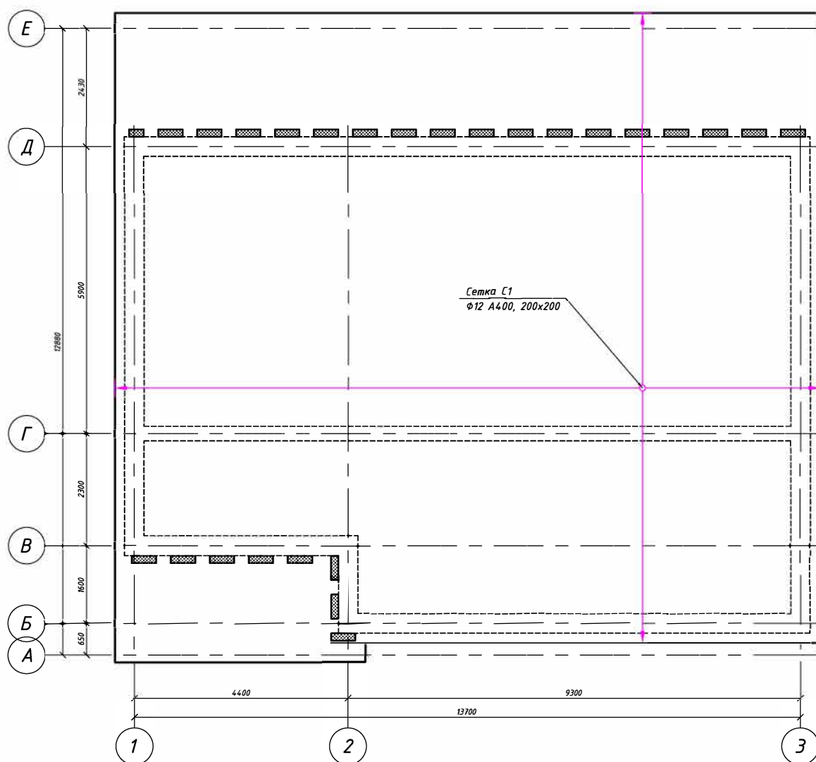
План армирования верхней и нижней сетки железобетонной плиты фундамента. (М1:80)
