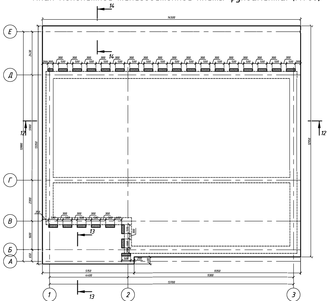
План монолитной железобетонной плиты фундамента. (М1:80)
