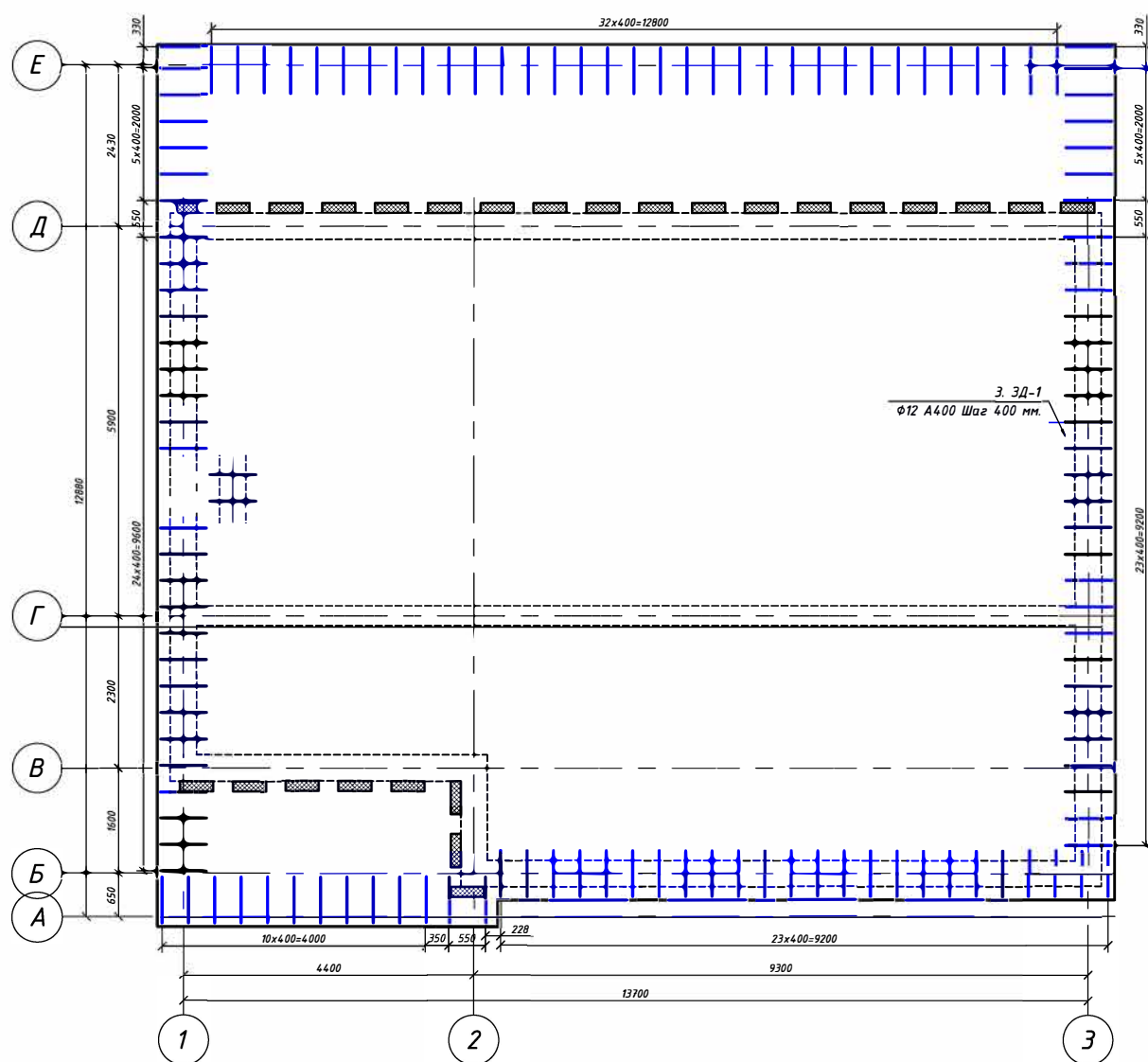
План закладных деталей фундамента. (М1:75)
