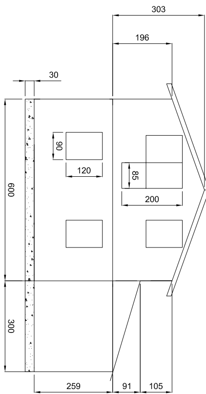
Фасада 1
