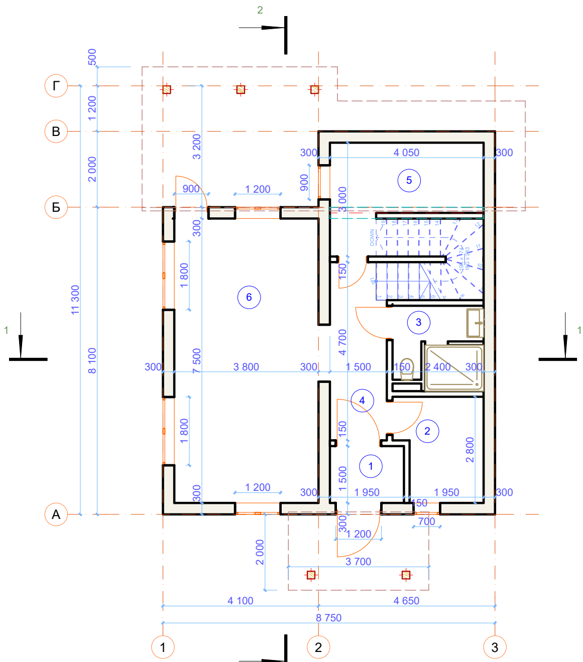
Экспликация 1-й этаж
