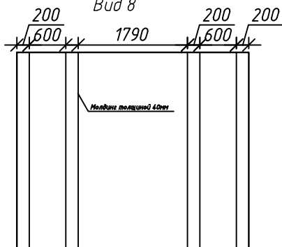
Вид 8
