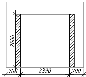
Вид 8.1
