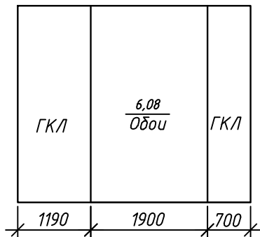
Вид 6
