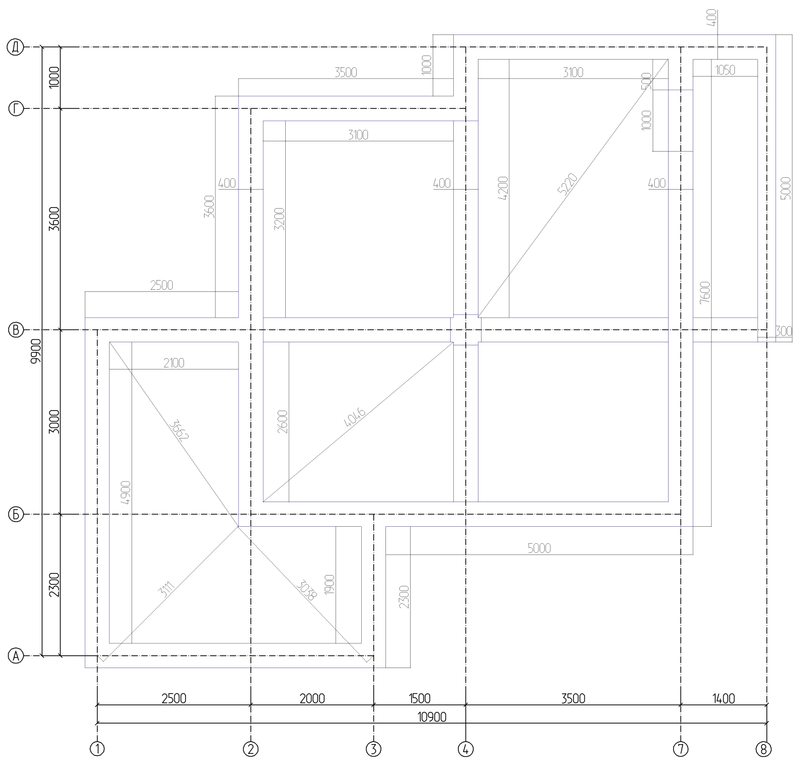
План фундамента
