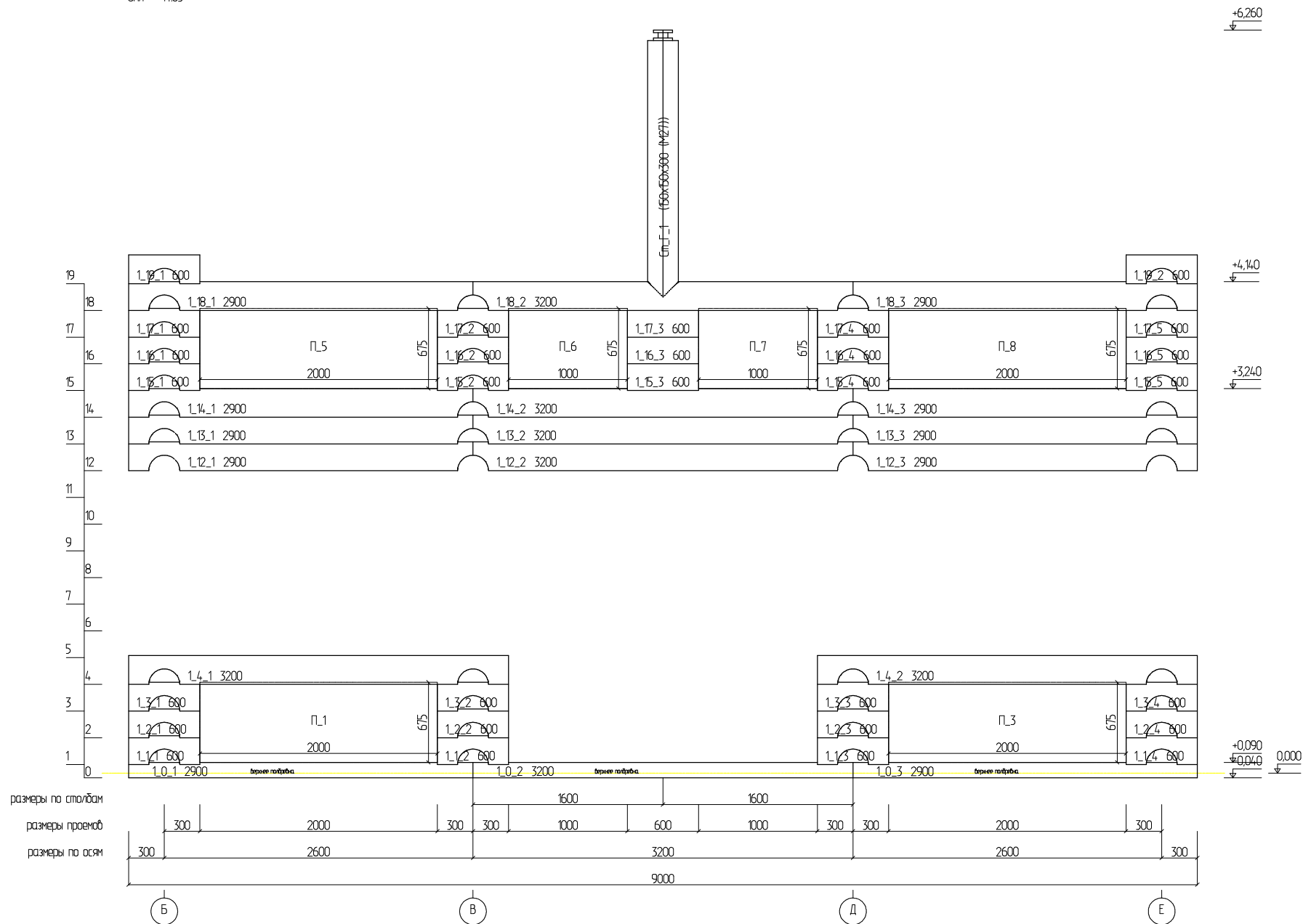
Развертка по стене (оси) 1
