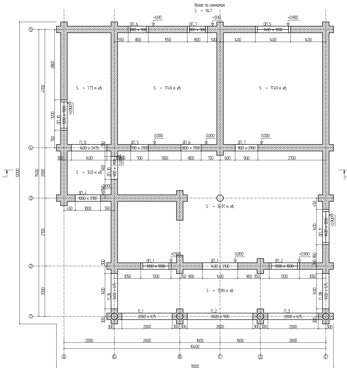
План на отн. 0,000
