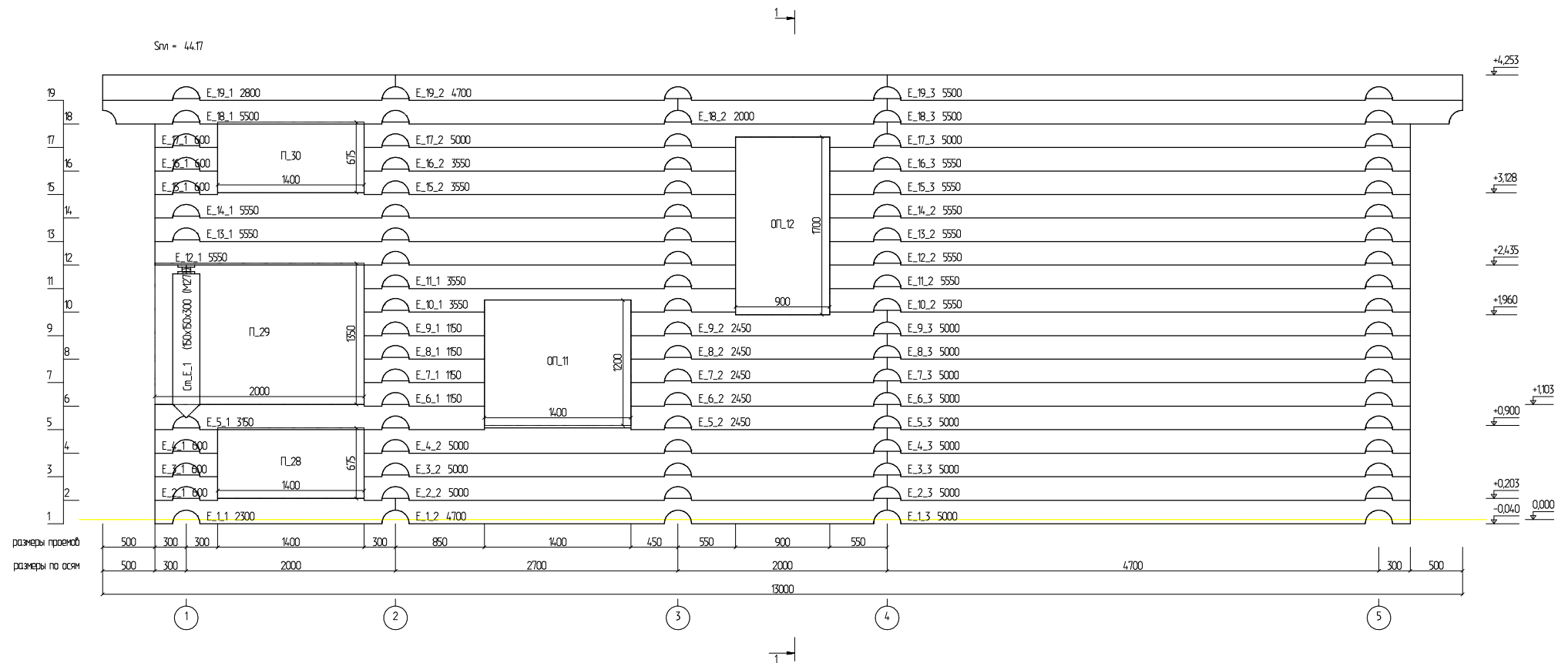
Развертка по стене (оси) Е
