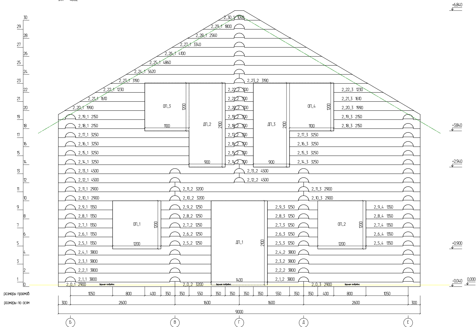
Развертка по стене (оси) 2
