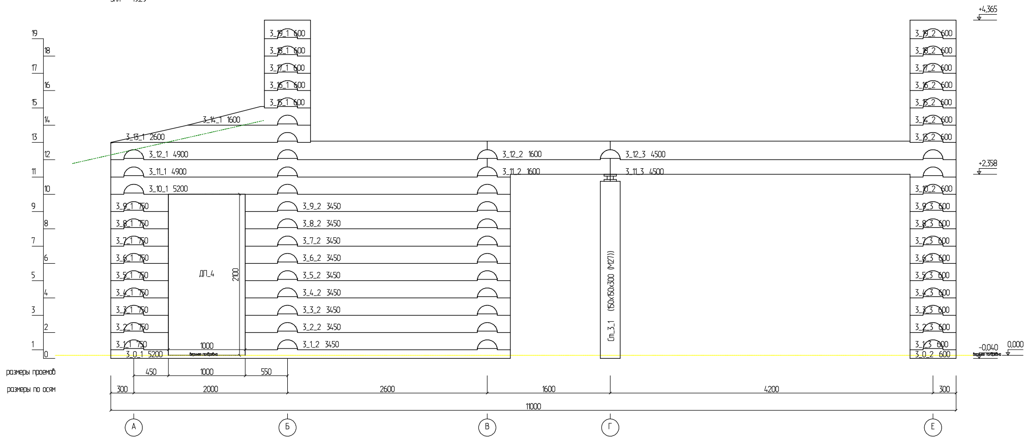
Развертка по стене (оси) 3
