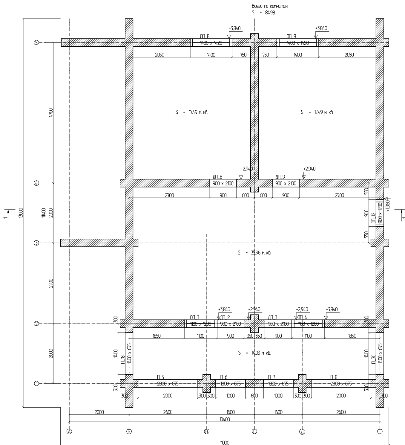
План на отм. +2,940
