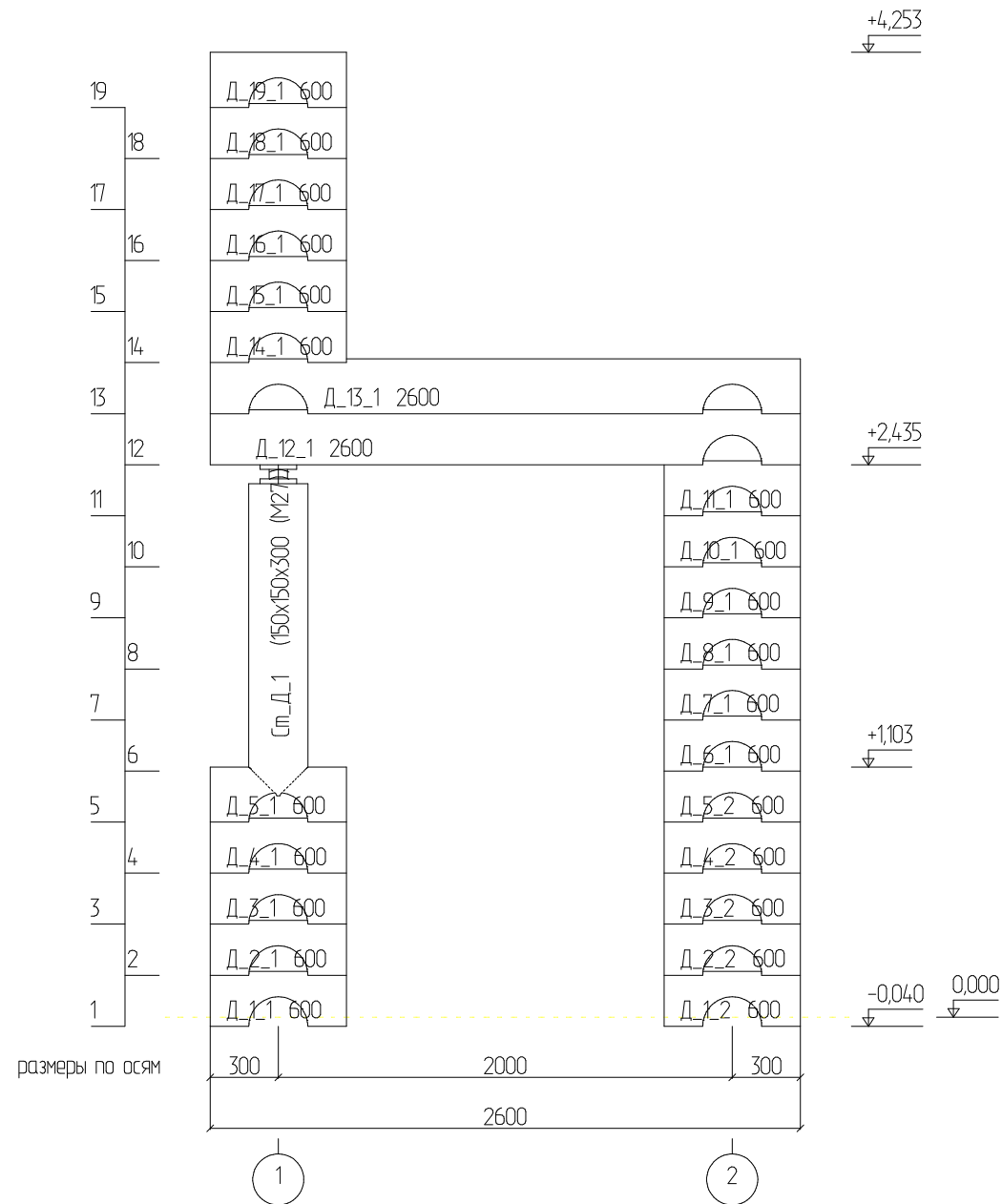
Развертка по стене (оси) Д
