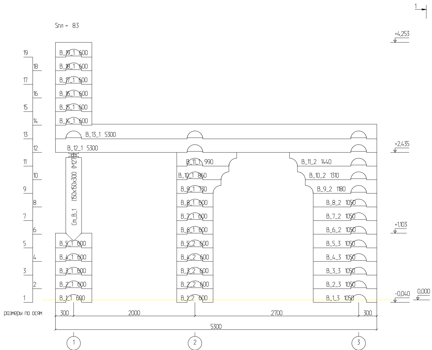
Развертка по стене (оси) В
