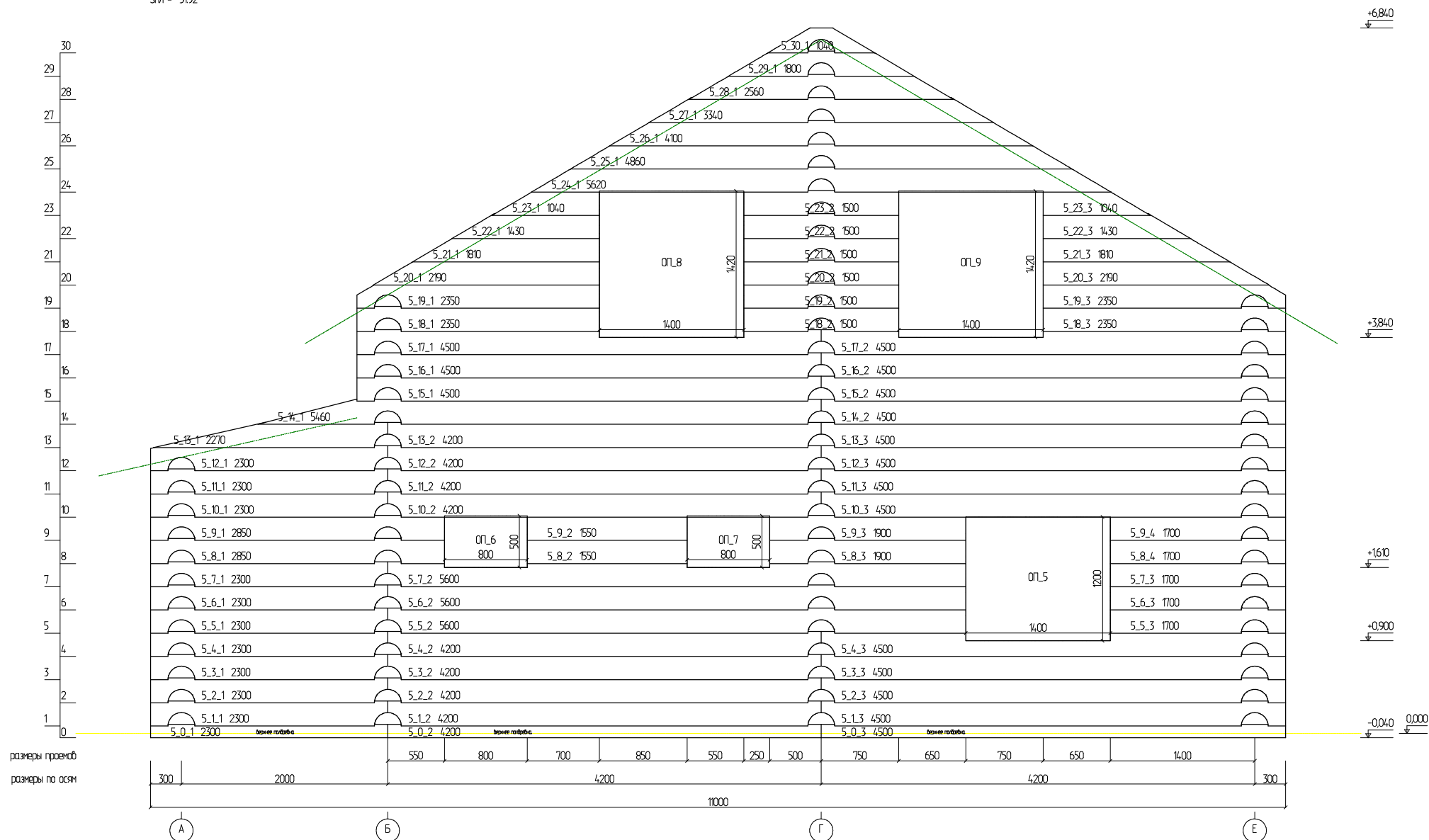
Развертка по стене (оси) 5
