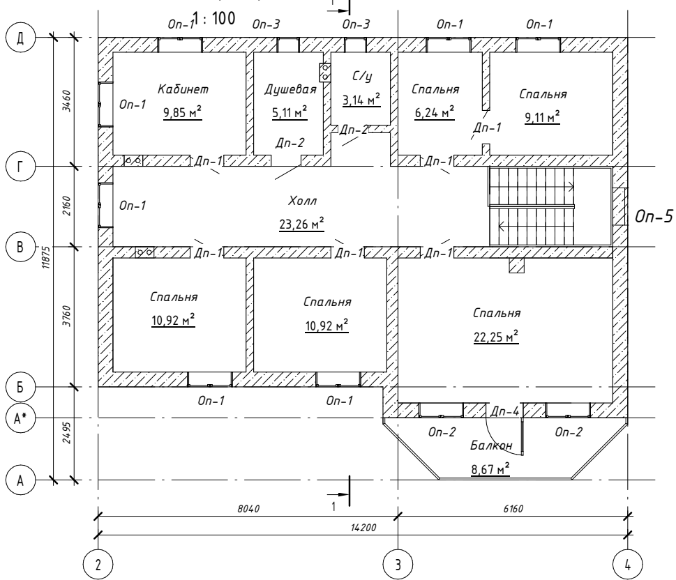
Маркировочный план 2 этажа
