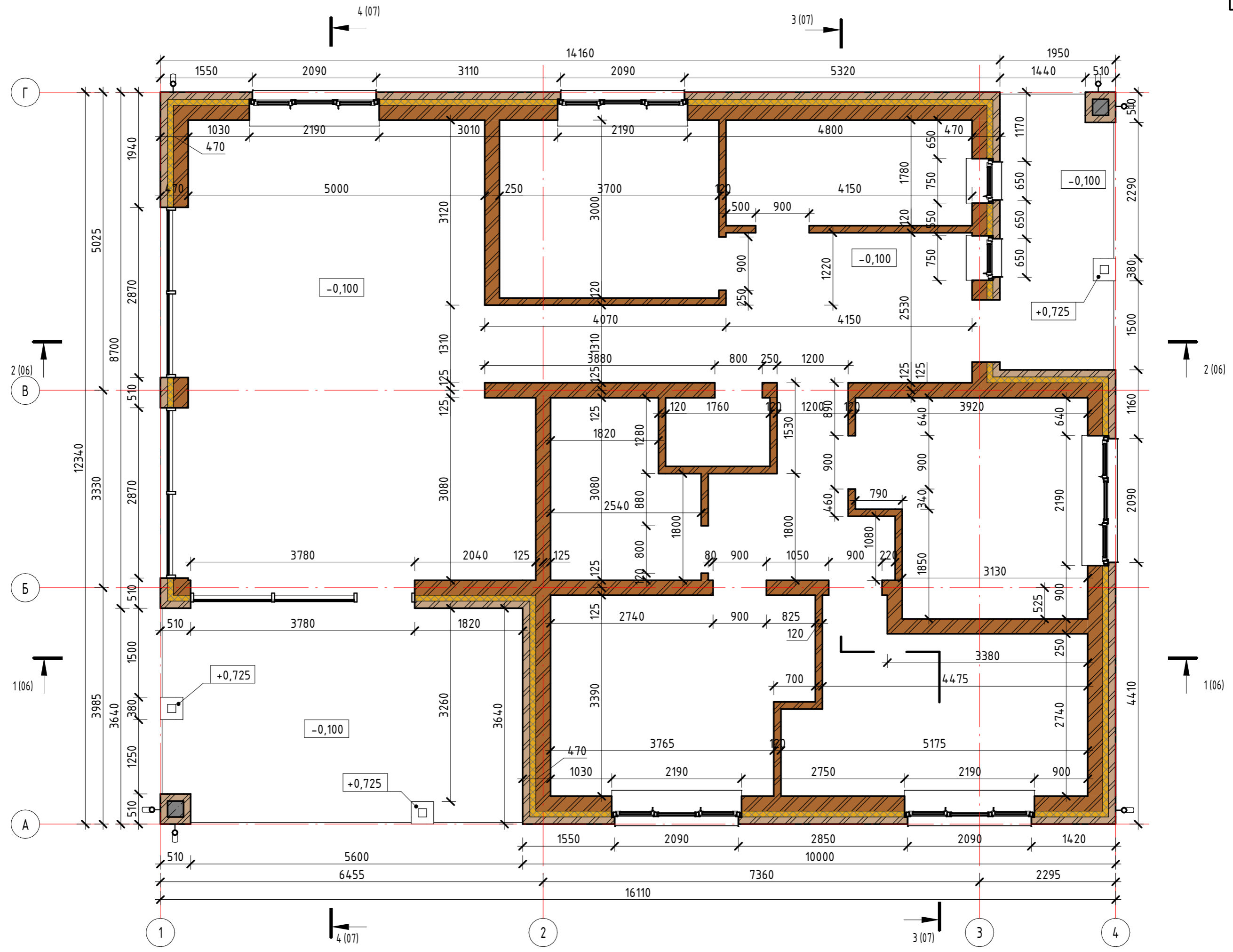
Кладочные план
