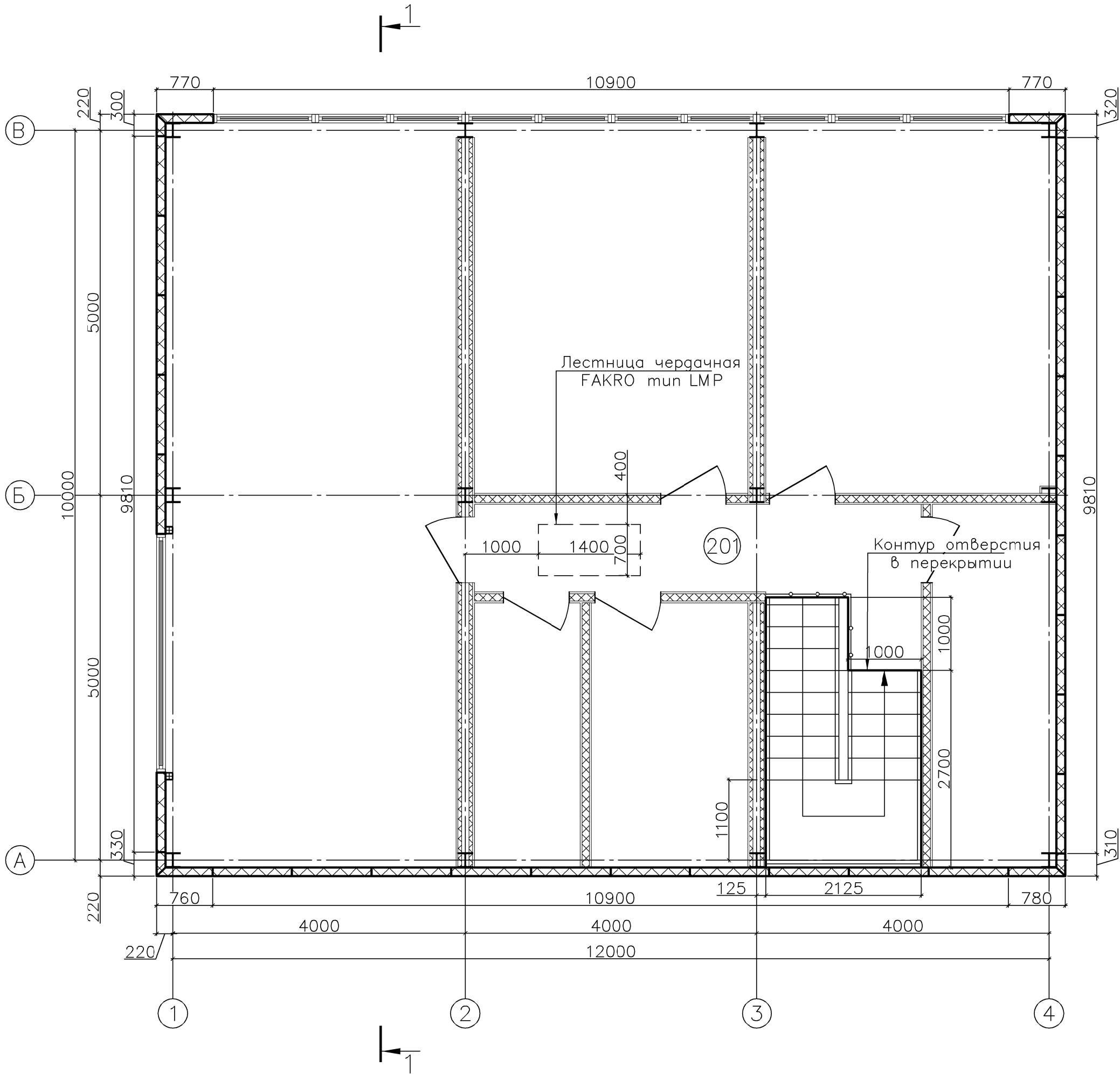
План на отм. +3,000
