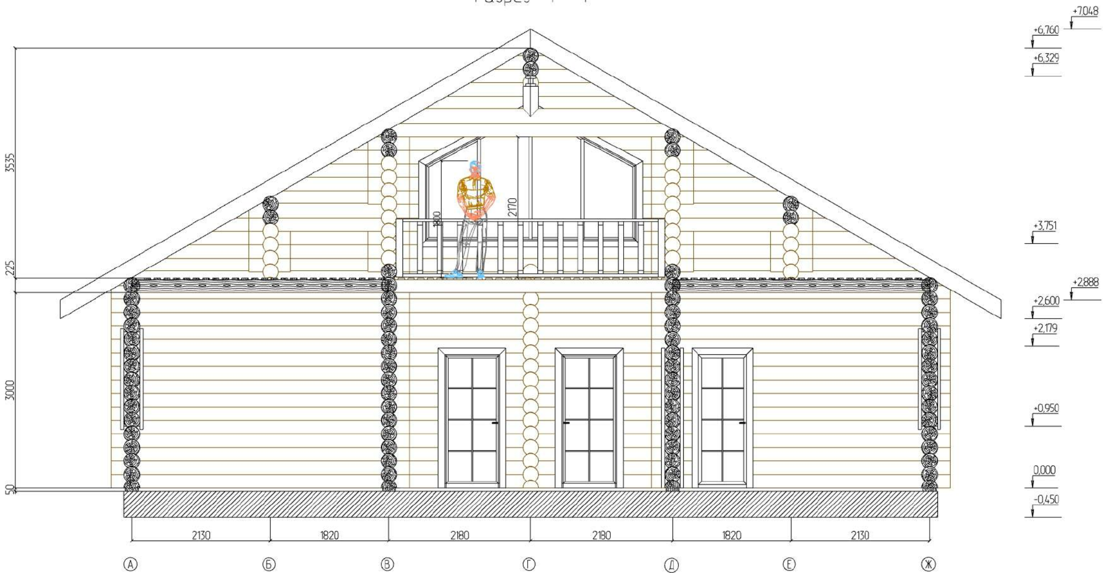
Разрез 1 - 1
