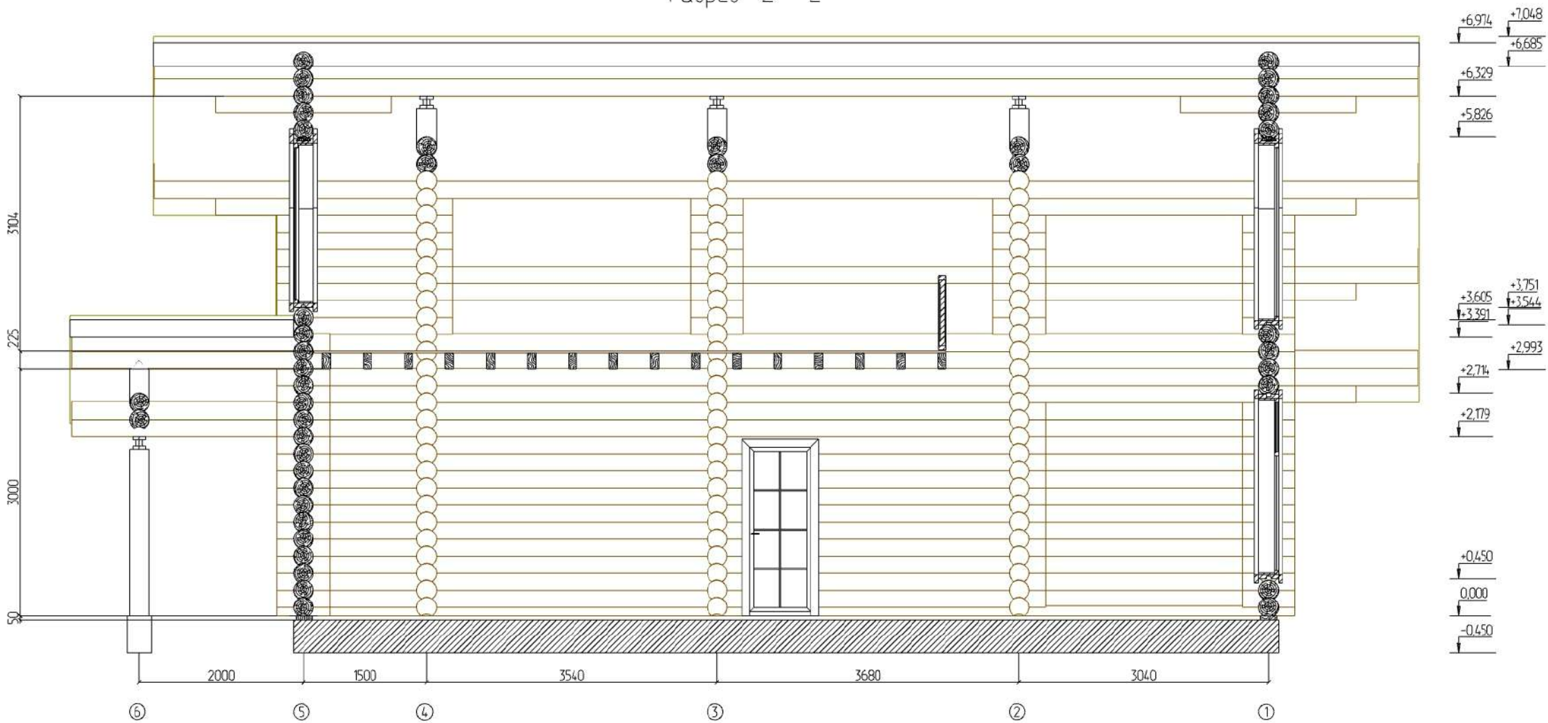
Разрез 2 - 2
