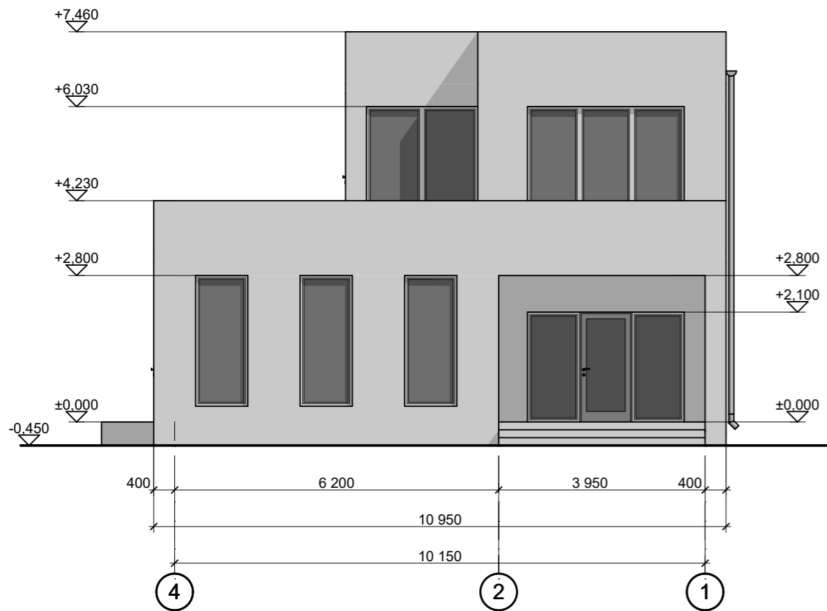
Фасад в осях 4 - 1
