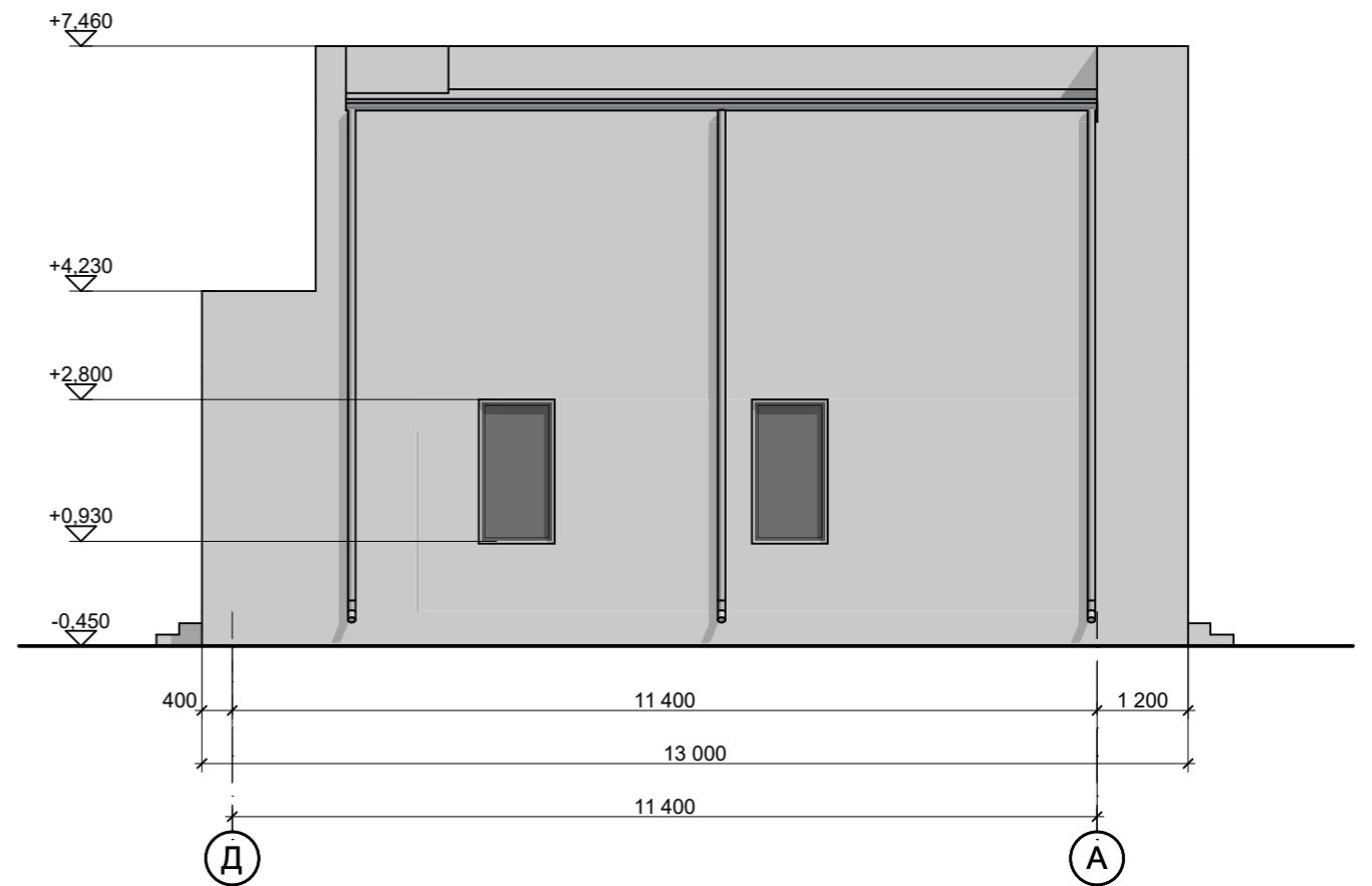
Фасад в осях Д - А
