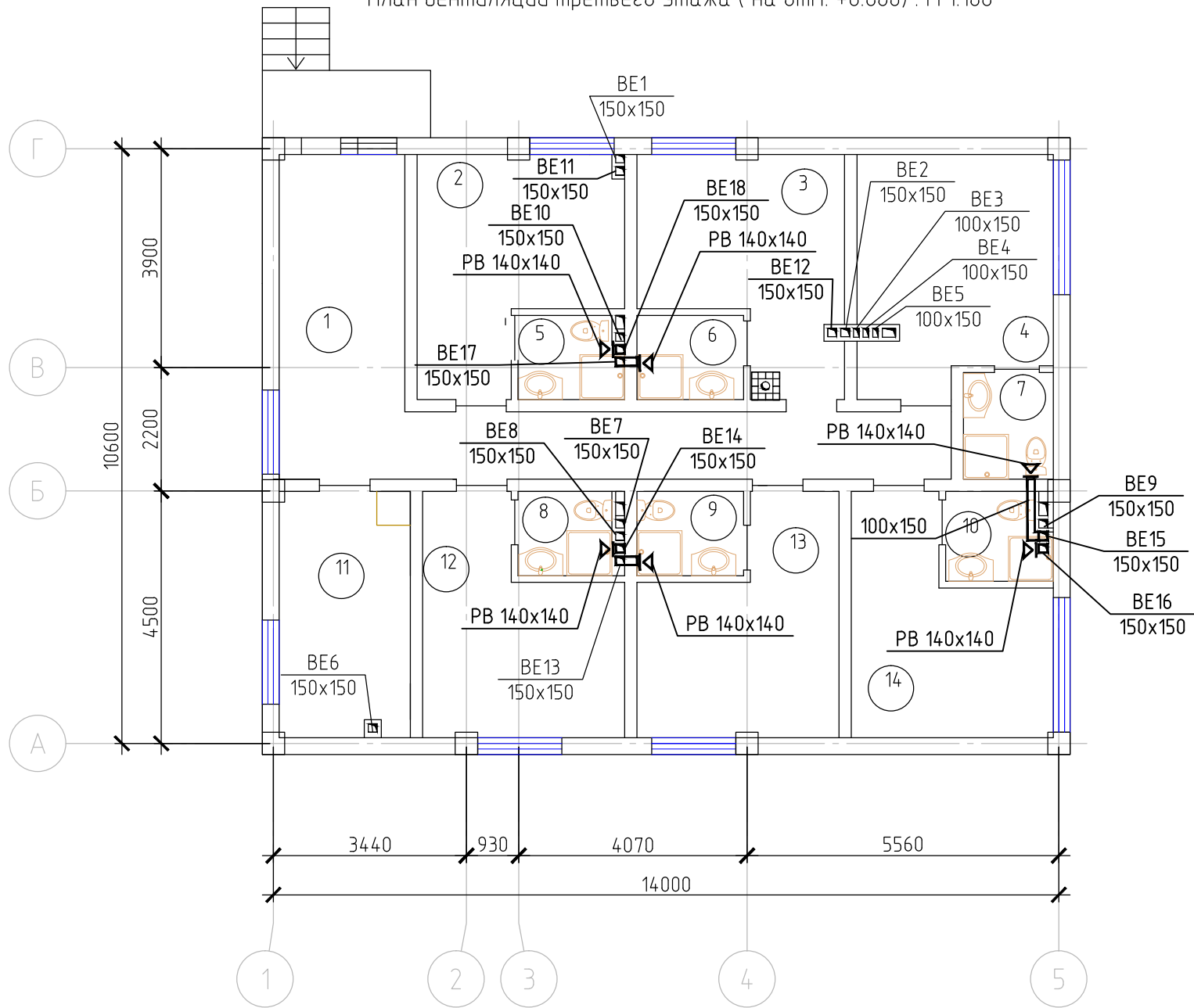
План вентиляции третьего этажа ( на отм. +6.600) . М 1:100
