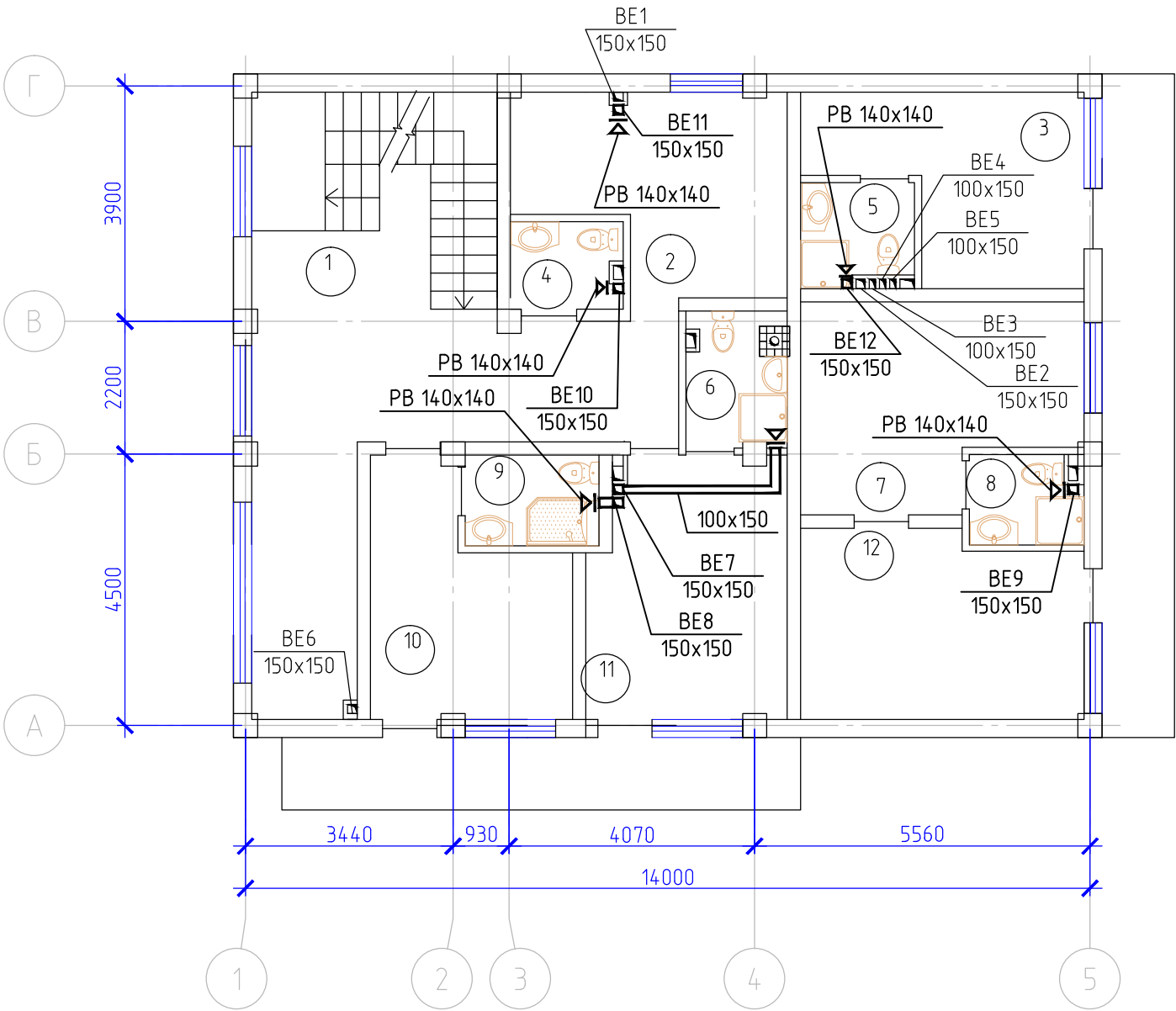
План вентиляции второго этажа ( на отм. +3.400). М 1:100
