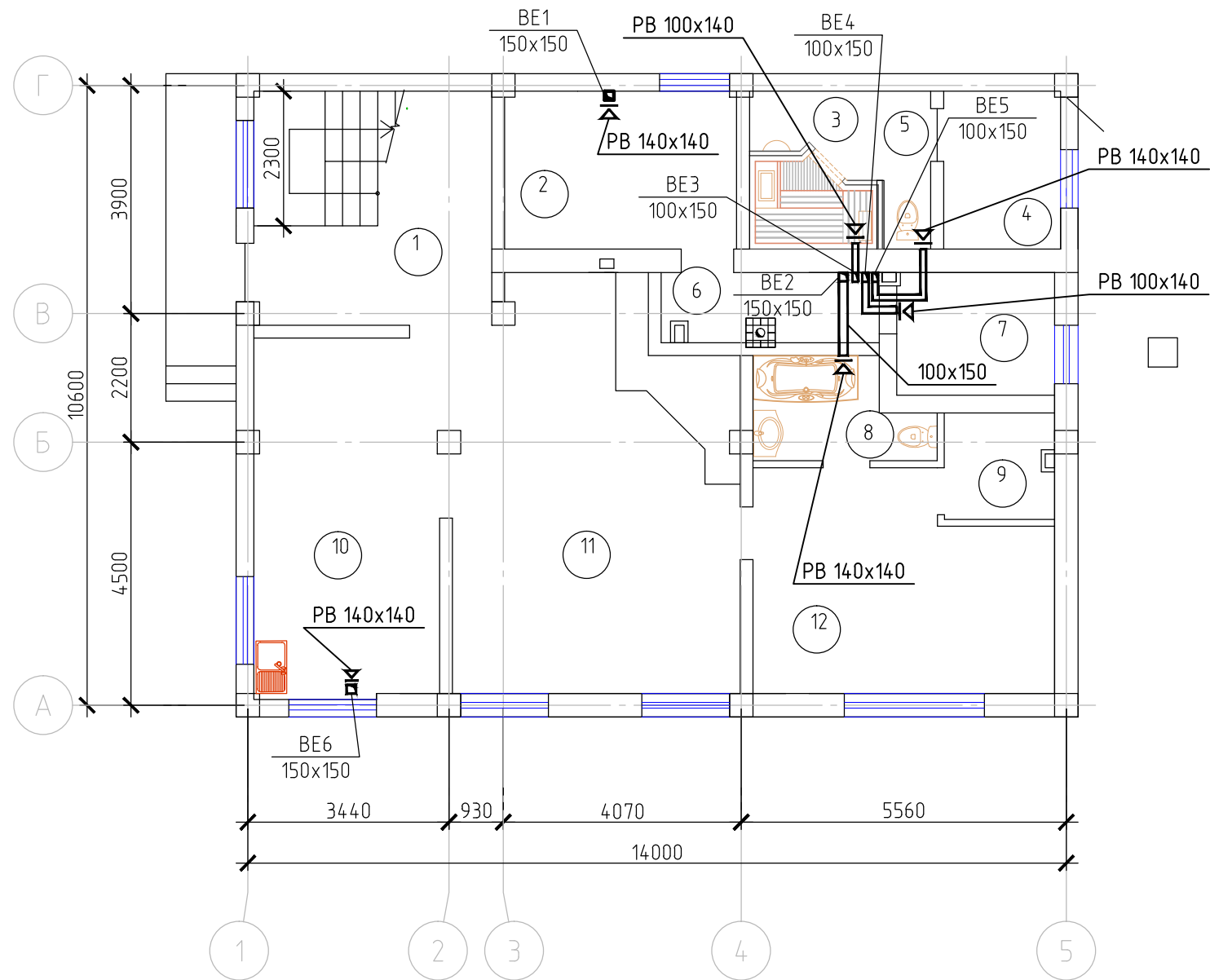
План вентиляции первого этажа ( на отм. 0.000). М 1:100
