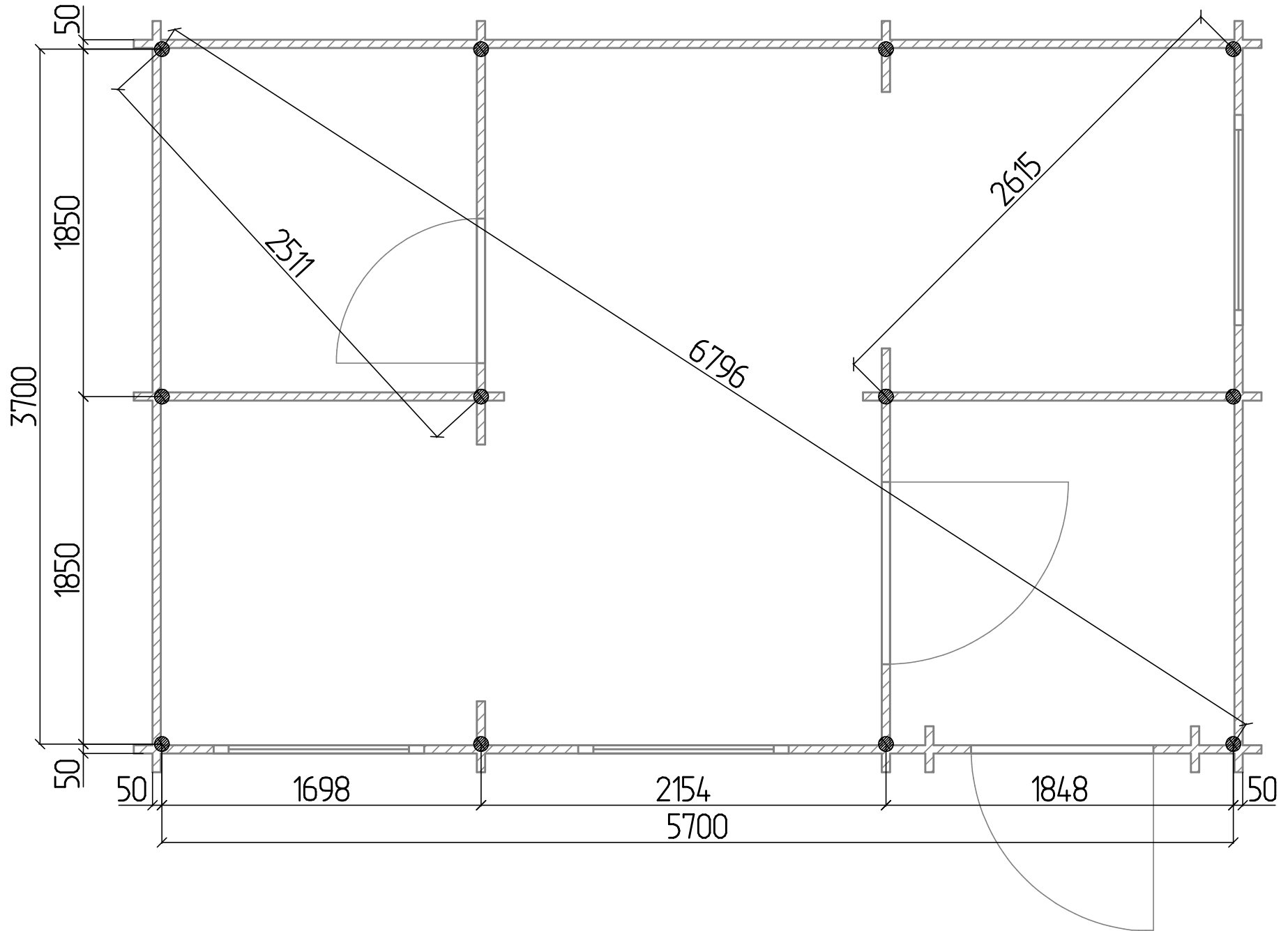
План свайного поля ДД336 габариты строения 4 x 6
